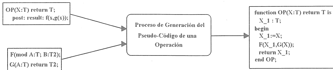
Figura 9.- Entradas y salidas del proceso de generación de código de la operación OP
