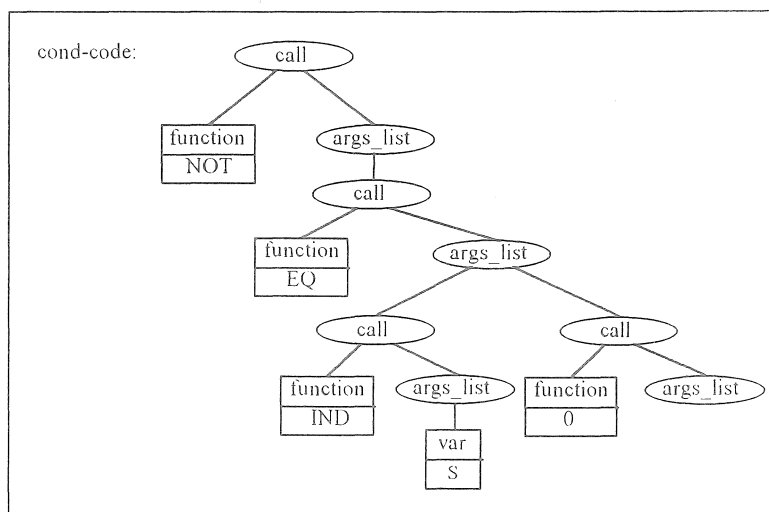
Figura 12.- Forma interna del código generado asociado a la precondición de la operación FIRST
