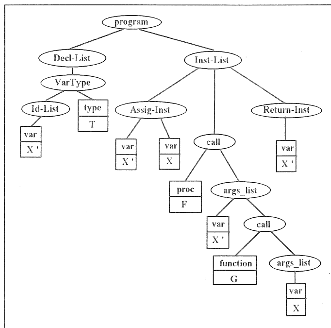
Figura 10.- Forma interna del código generado
