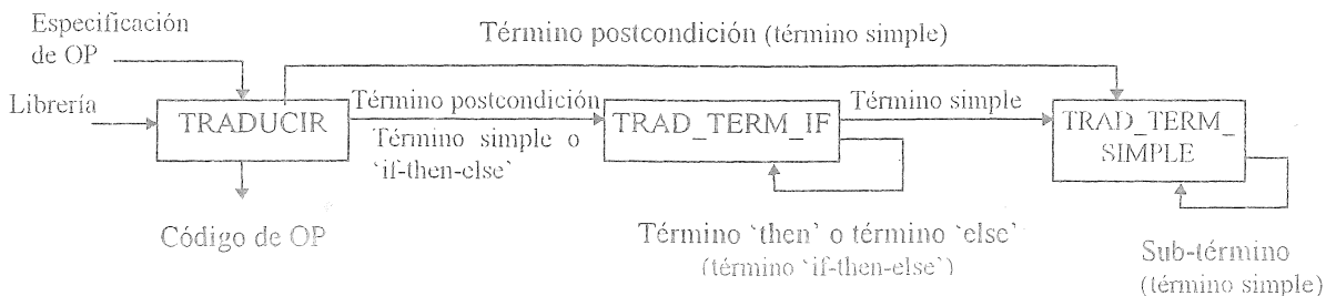
Figura 8.- Flujo de datos entre las funciones que generan el código de una operación
