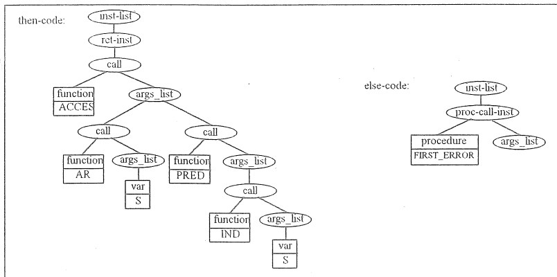
Figura 13.- Forma interna del código asociado a la postcondición y a la excepción de la precondition
