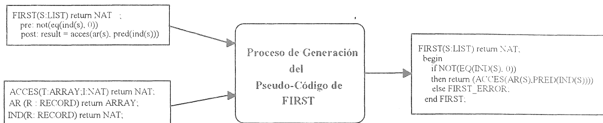
Figura 11.- Entradas y salidas del proceso de generación de código de la operación FIRST
